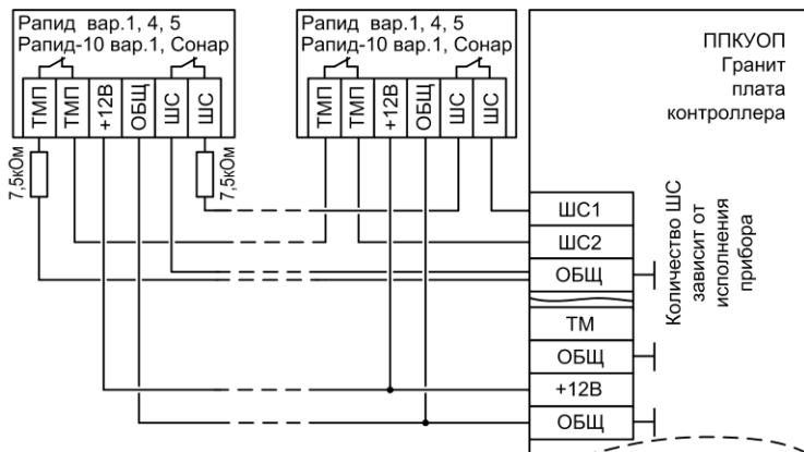
Рис.Б3 Схема подключения охранных извещателей Рапид вар.1,4,5, Рапид-10 вар.1, Сонар (тампер подключён к отдельному ШС)
