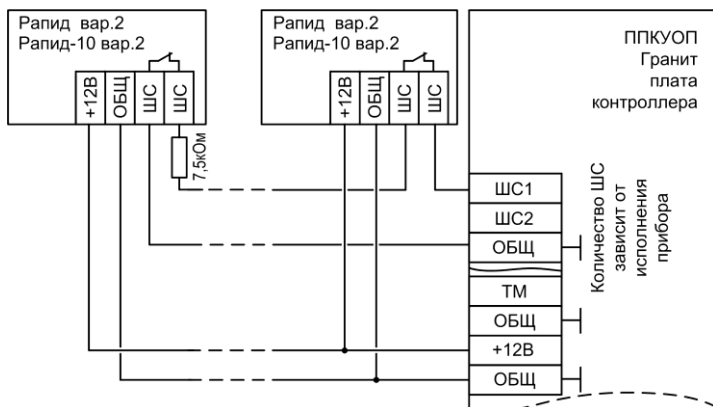
Рис.Б4 Схема подключения охранных извещателей Рапид вар.2, Рапид-10 вар.2
