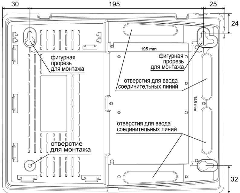
Рис.3 Задняя стенка прибора. Присоединительные размеры
