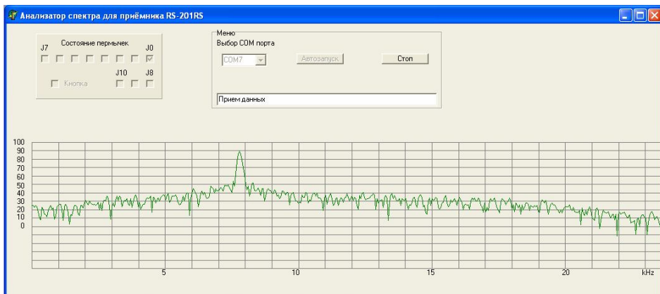
Рис. 4. Программа «Анализатор»
