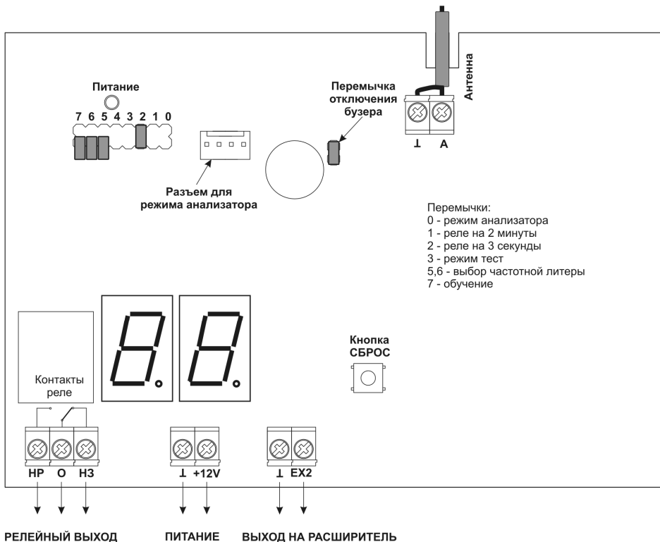
Рис. 5. Монтажная схема приёмника
