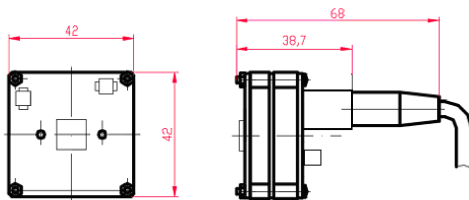
Рис.6а. Размеры.
