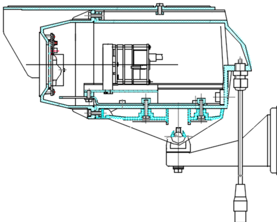
Рис.3б. Стандартный корпус.
