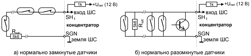
Рис. 5 – Примеры монтажа охранных шлейфов
