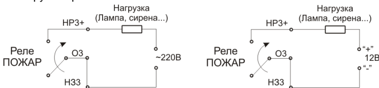
Рис. 1 – Примеры подключения нагрузки к реле ПОЖАР
