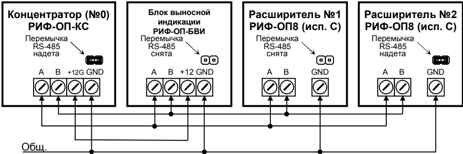
Рис. 7 – Пример подключения расширителей к концентратору
