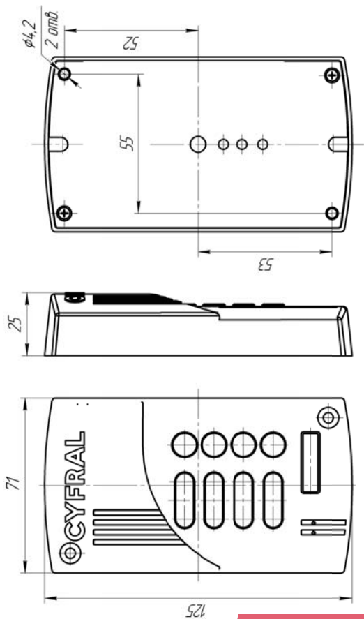
Рисунок А.2 Установочные и габаритные размеры блока вызова ЦИФРАЛ М-4.1М (ЦИФРАЛ М-4.1М/У, ЦИФРАЛ М-4.1М/УС)
