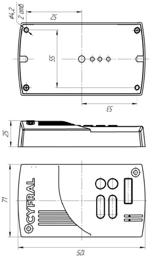
Рисунок А.1 Установочные и габаритные размеры блока вызова ЦИФРАЛ М-2.1М (ЦИФРАЛ М-2.1М/У, ЦИФРАЛ М-2.1М/УС)
