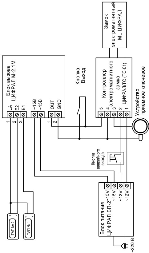
Рисунок Б.1 Схема подключения домофона ЦИФРАЛ М-2.1М
