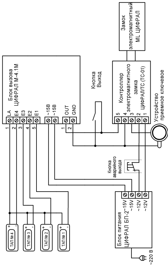
Рисунок Б.3 Схема подключения домофона ЦИФРАЛ М-4.1М
