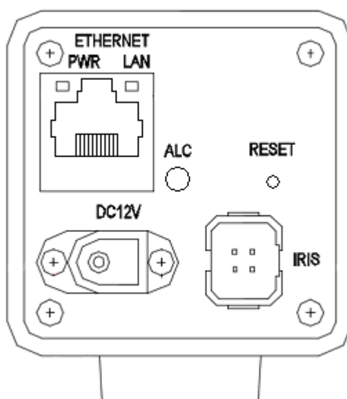
Рис.16. Камера VEC-157-IP
