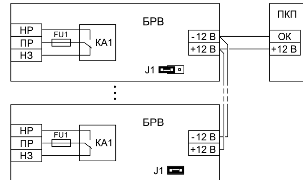
Рис.5 Схема подключения нескольких БРВ к выходу ОК ПКП, контроль СЛ до последнего БРВ
