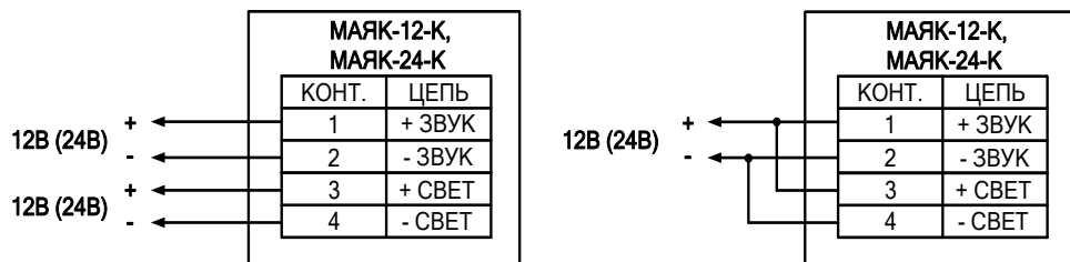
Рис. 1. Схема подключения.
