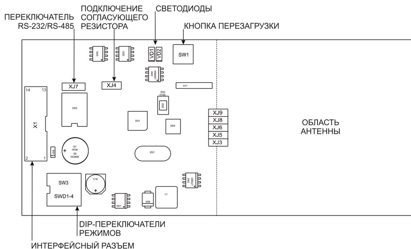
Рисунок 2. Схема печатной платы считывателя
