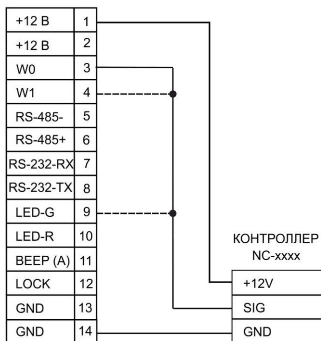
Рисунок 3. Схема подключения по протоколу Parsec, адрес 1
