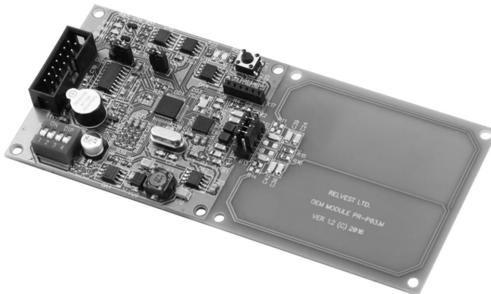
Рисунок 1. Считыватель PNR-P03E
