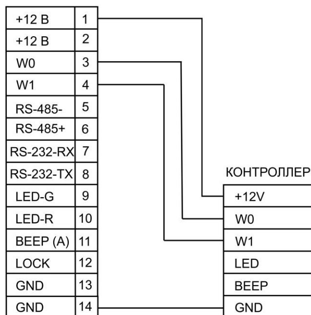
Рисунок 4. Схема подключения по протоколу Wiegand
