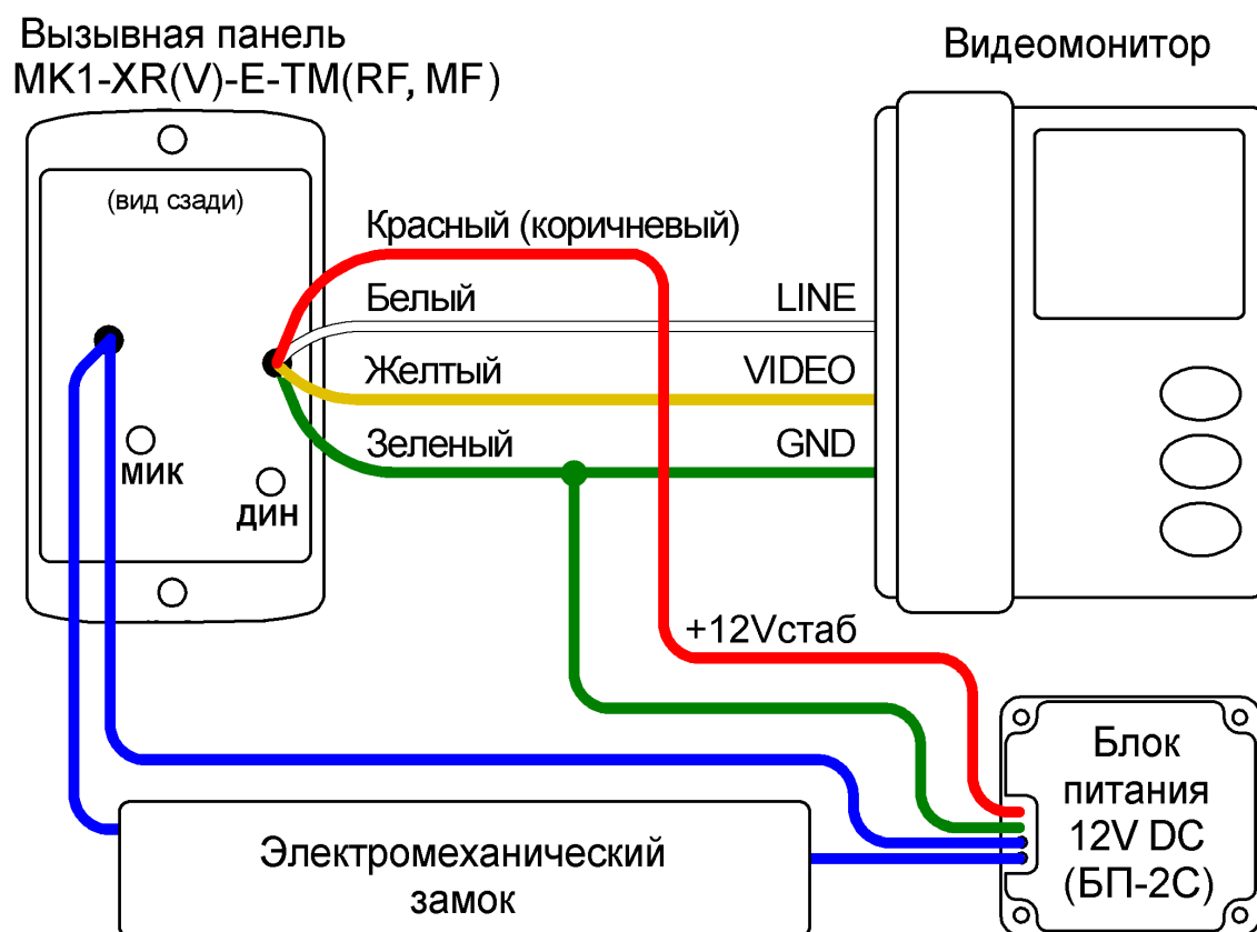
Рис 2. Подключение блока вызова MK1-XRV-E-TM(RF, MF)
