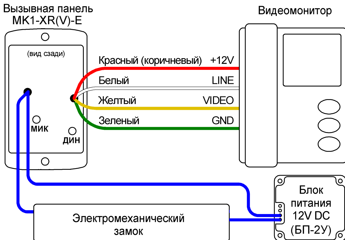
Рис 1. Подключение блока вызова MK1-XRV-E
