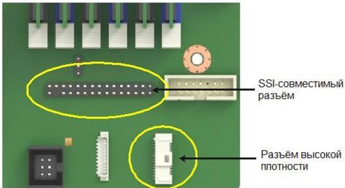
Рисунок 50. Варианты разъемов
