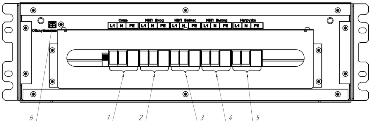
Рисунок 2 Габаритно-присоединительные размеры ББ. Вид сзади.
