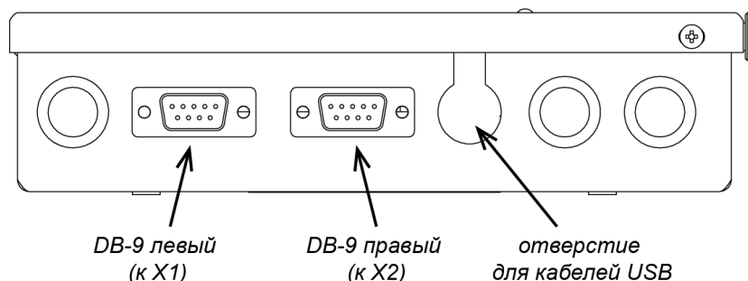
Рисунок 5. Расположение разъемов DB-9 (RS-232) на корпусе контроллера
