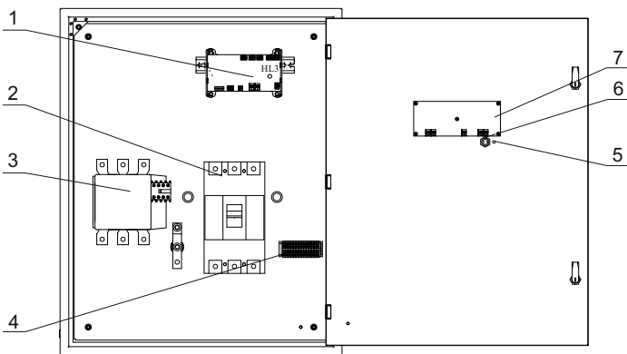
в) ШУН/В мощностью 55-110 кВт
