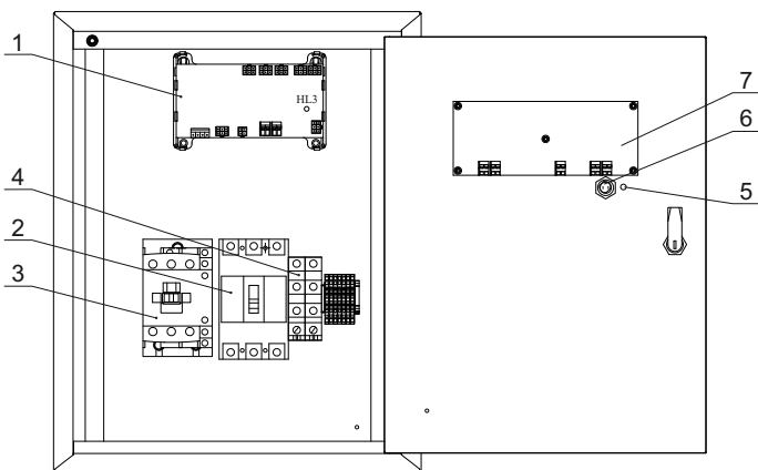
б) ШУН/В мощностью 18-45 кВт
