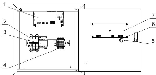
а) ШУН/В мощностью 0,18-15 кВт
