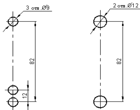
Рис1 Разметка под установку изделия
